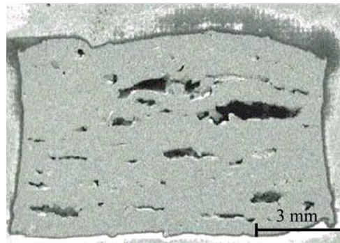
شکل ۵- شکل‌گیری حفره‌های ترک‌مانند در نمونه‌ی تولید شده در سیکل عملیات حرارتی ۶۶۰ °C / ۱۵ min
