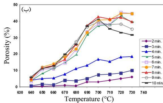
شکل ۹- تغییرات (الف) چگالی و (ب) درصد تخلخل فوم‌های تولید شده بر حسب دمای فوم‌سازی در زمان‌های نگهداری متفاوت
