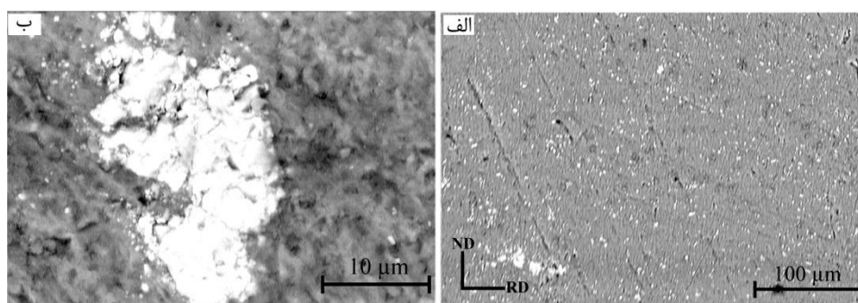
شکل ۳- الف) تصویر SEM در جهت RD/ND پیش‌فرم تولید شده
