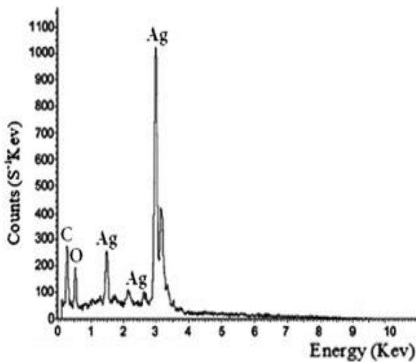
شکل ۷- آنالیز عنصری EDX نانو ذرات
