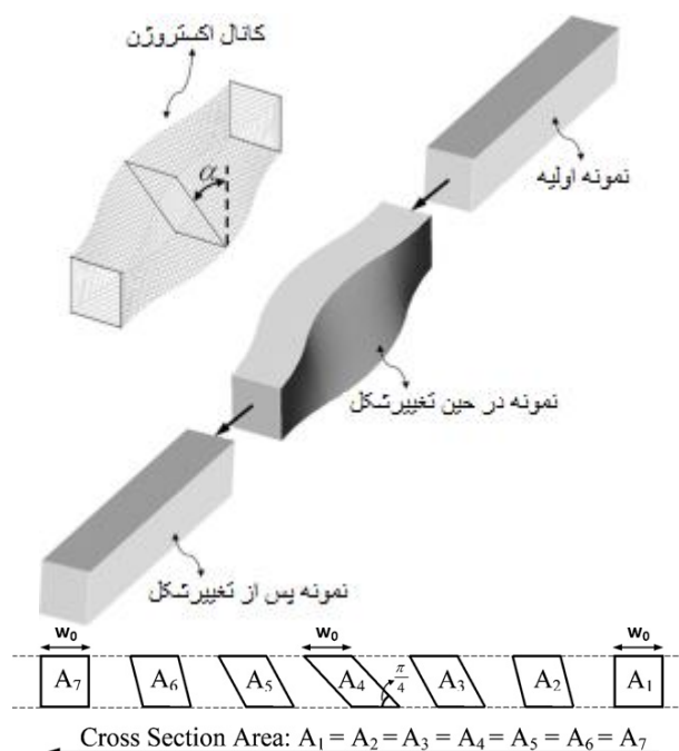
شکل ۱. نمایش شماتیک از فرایند اکستروژن برشی ساده و نحوه تغییر شکل ماده [۸].
