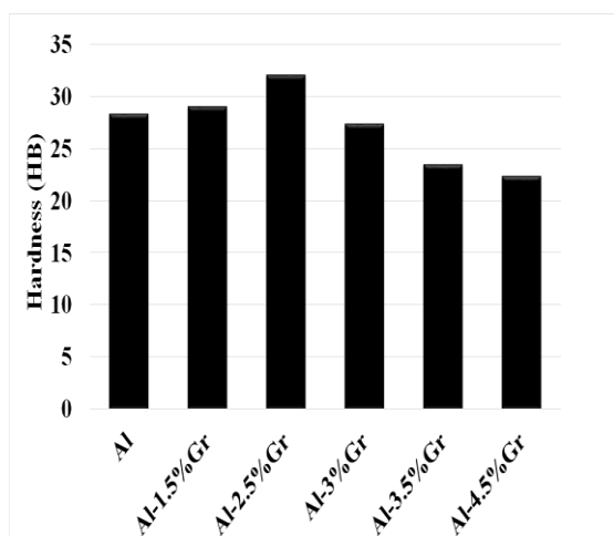
شکل ۱۱ - نمودار سختی کامپوزیت Al-Gr با
