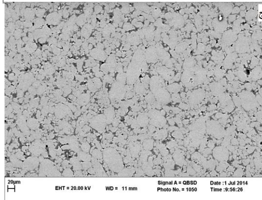
شکل ۵ - تصویر SEM کامپوزیت‌های الف - Al - 4.5 % Gr - ب - Al - 3 % Gr - ج - Al - 1.5 % Gr - د - Al - 2.5 % Gr تولید شده به روش همگن سازی در مایع-پرس سرد-تف جوشی در کوره خلأ
