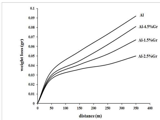
شکل ۶ - نمودار سایش کامپوزیت Al-Gr با درصدهای مختلف گرافیت و آلومینیم خالص تولید شده به روش همگن سازی در مایع-پرس سرد-تف جوشی در کوره خلأ
