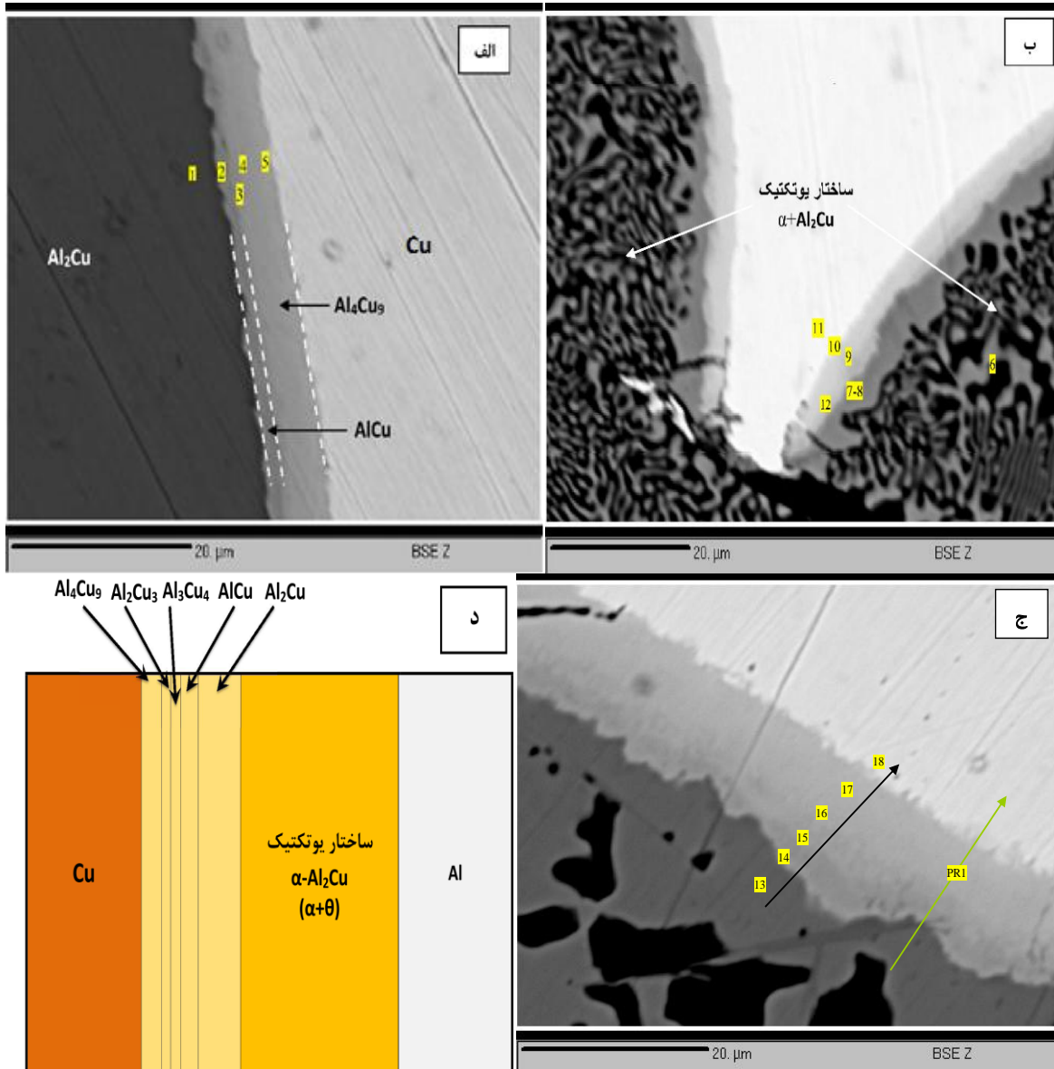
شکل ۳- الف) لایه مجاور مس در فصل مشترک نمونه A700C25 (ب) بخشی از لایه فصل مشترک نمونه A700C40 (ج) قسمتی از فصل مشترک نمونه A800C220 (د) شکل شماتیکی فصل مشترک
